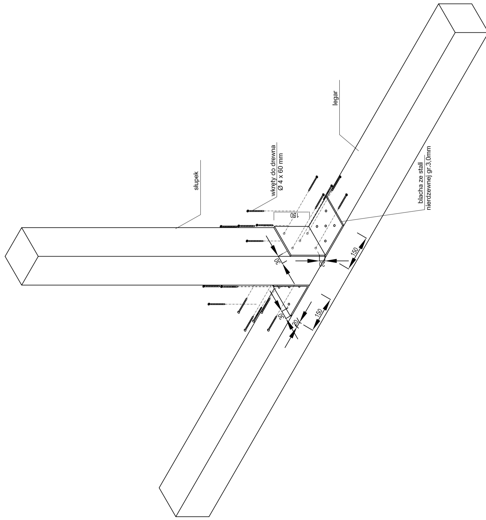
Mocowanie słupków do legarów skala 1:10
