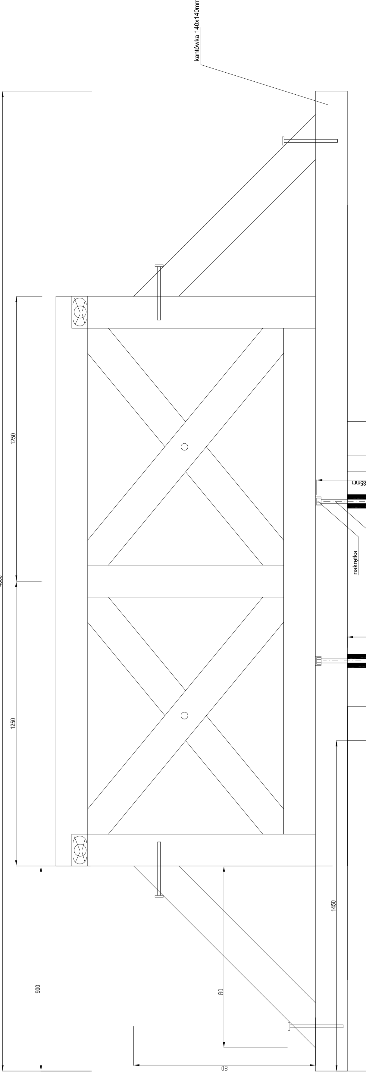
Mocowanie legarów do podłoża betonowego skala 1:10
